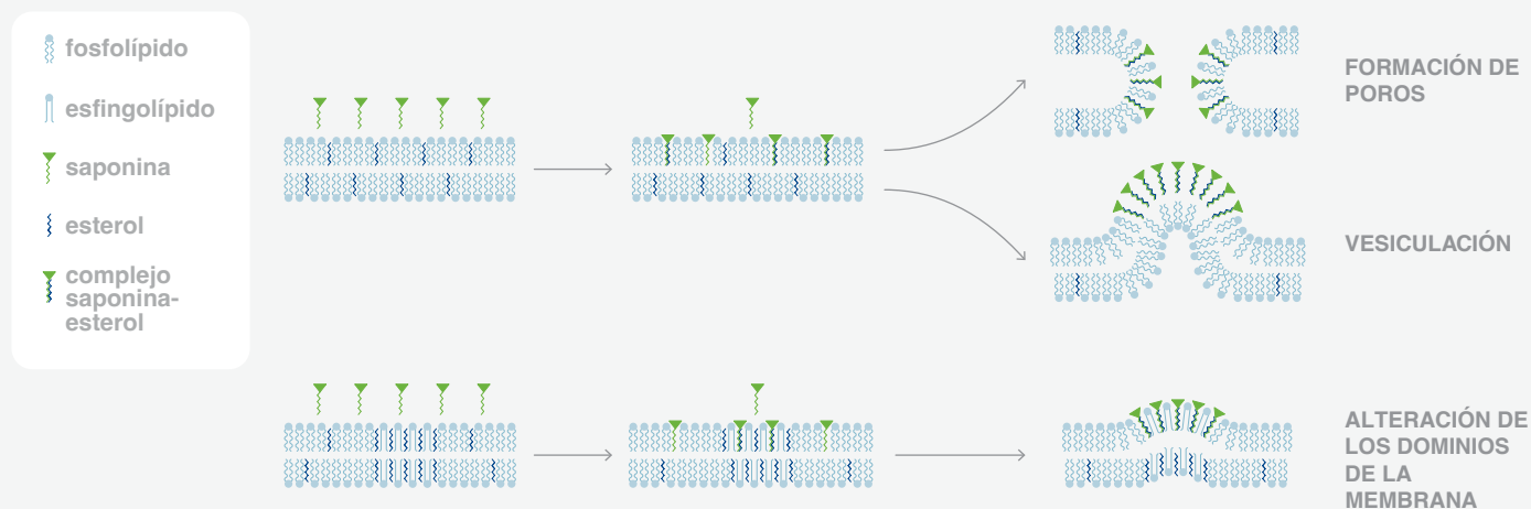
Figura 4. Las saponinas de Quillaja interactúan con el colesterol en la membrana celular, modulando su plasticidad mediante la inducción de la formación de poros, la vesiculación y la alteración de los dominios de la membrana. Este mecanismo reduce las tasas de infección celular y mejora la absorción de nutrientes (adaptado de Augustin et al. 2011).
