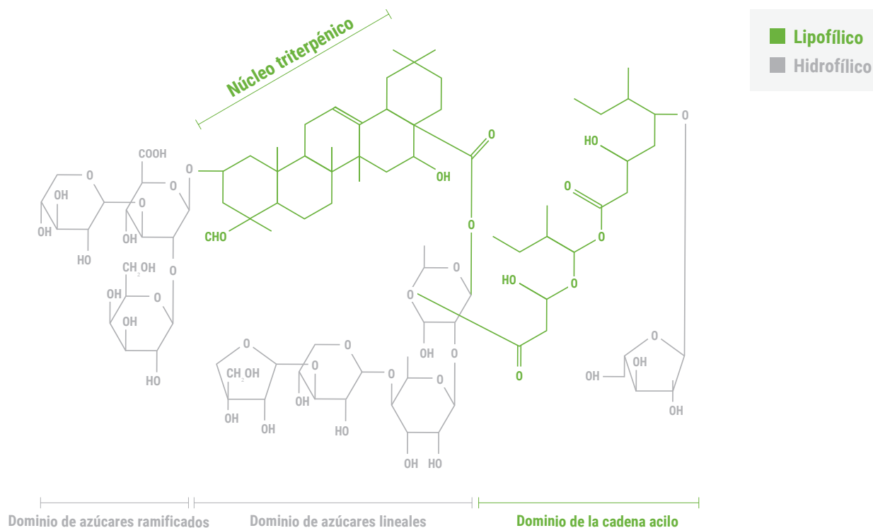
Figura 1. Estructura general de la molécula de saponina, que muestra las regiones hidrofílica y lipofílica responsables de la actividad de superficie de la molécula (adaptado de Yang et al. 2013).
